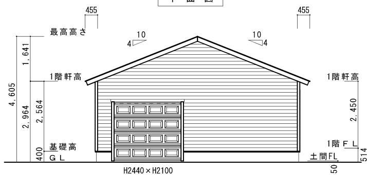
A側立面図
