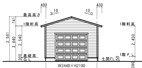
A側立面図
