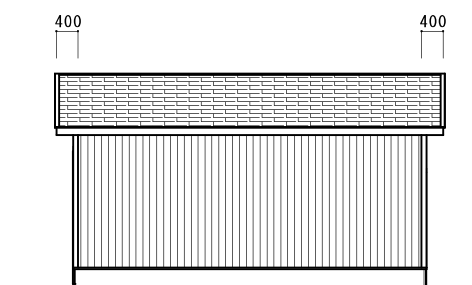
D 立面図
