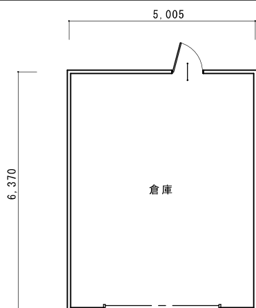
平面図
