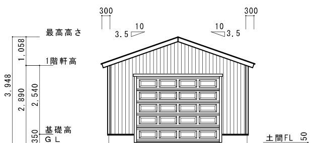
A 立面図
