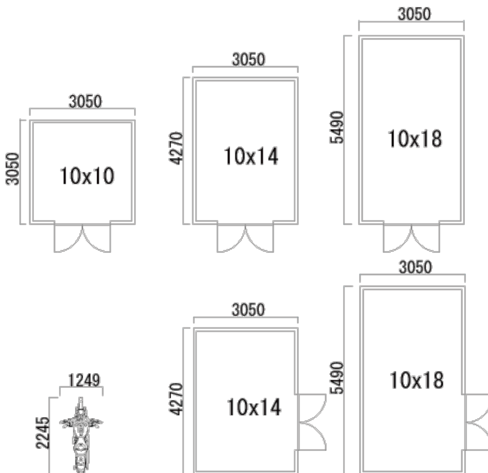
パークレー平面図(バイクガレージ・物置・趣味の工房等)
