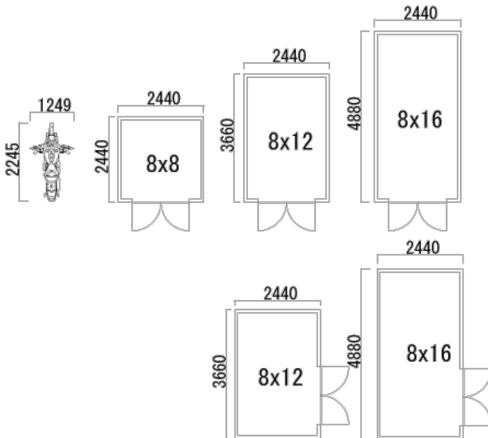
ブラッドフォード平面図(バイクガレージ・物置・趣味の工房等)
