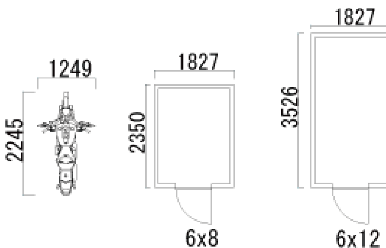
キャスパー平面図(物置・キッズハウス等)
