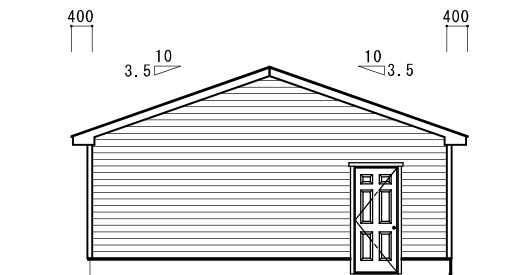
B側立面図
