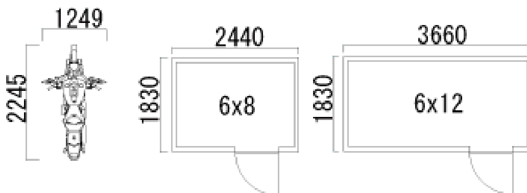
ランカスター平面図(物置・小屋等)
