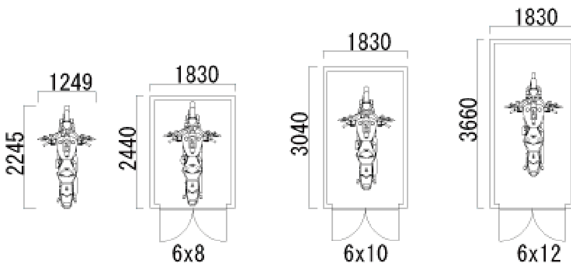
ランカスターバイクガレージ平面図(バイクガレージ・物置等)
