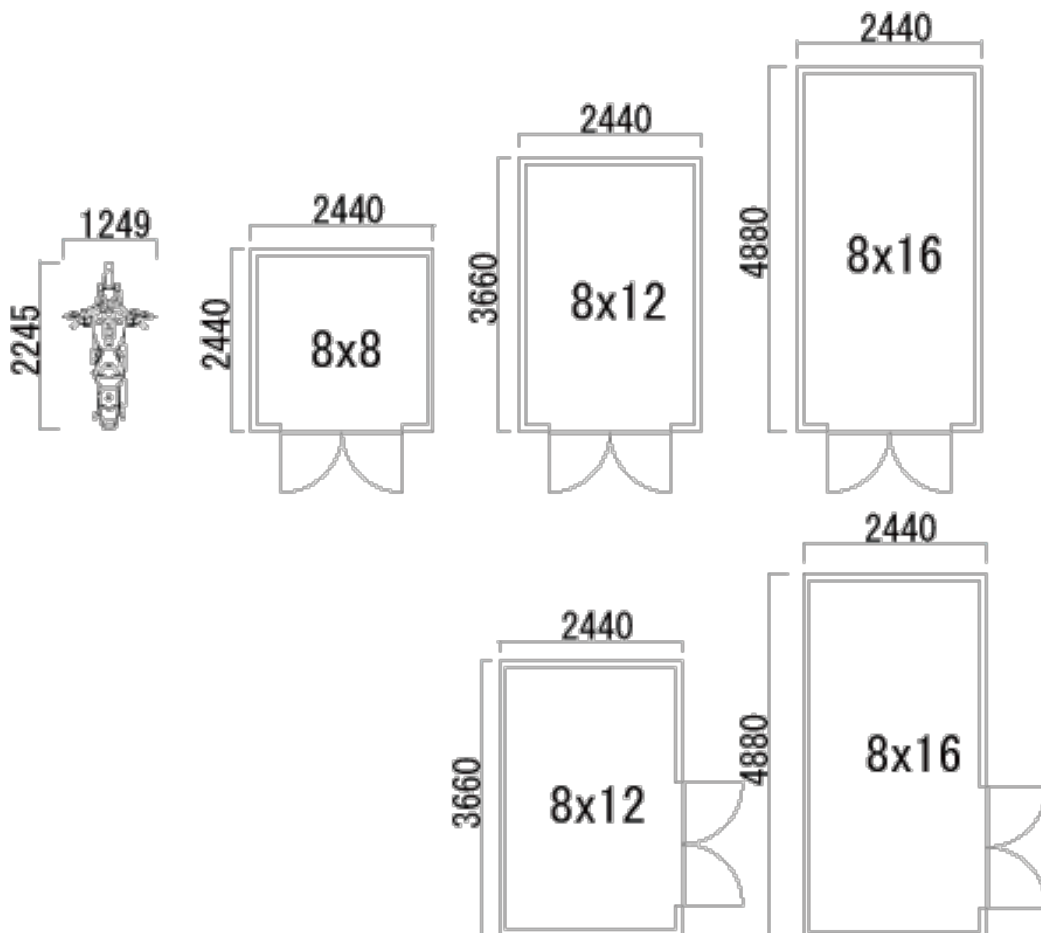
マジェステック平面図(バイクガレージ・物置・趣味の工房等)
