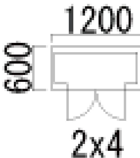
サイドボックス平面図
